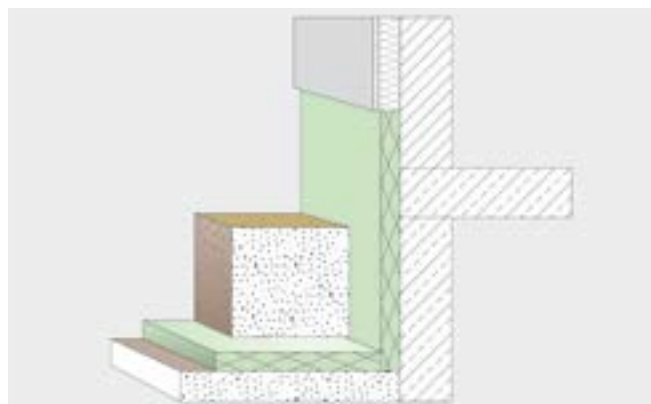
Fig. 5: La protezione antigelo viene posata sotto alla linea di gelo nel terreno.
