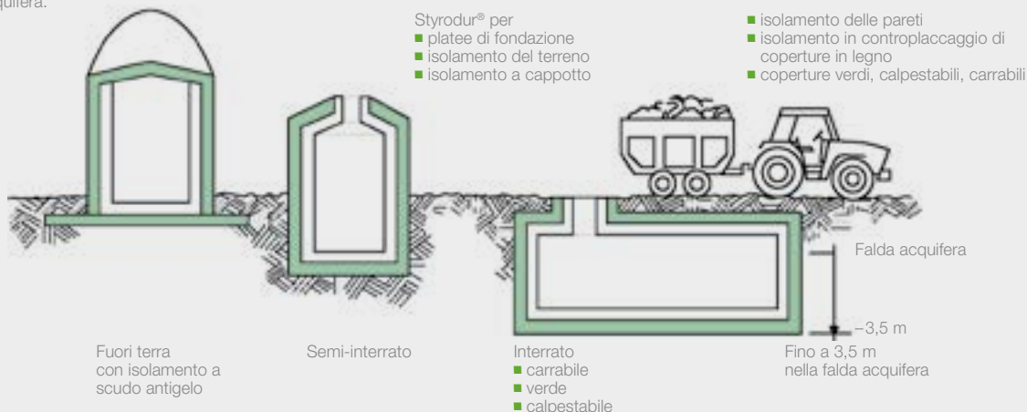
Fig. 3: Isolamento termico con Styrodur® di differenti tipologie di fermentatori.
