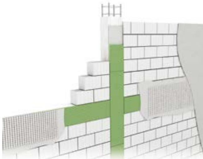
Fig. 1: Isolamento di ponti termici trave/pillastro
