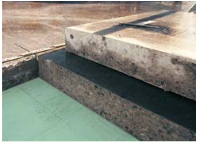
Fig. 52: Lastra della carreggiata in calcestruzzo gettato in opera per lo studio scientifico del comportamento nel lungo periodo.
