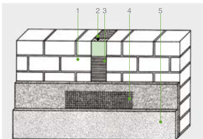
Fig. 20: Architrave della finestra nella muratura da isolare termicamente; stesura orizzontale dello strato adesivo per l'intonaco.
