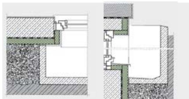
Fig. 22: Raccordo di un lucernario in calcestruzzo.
