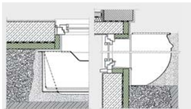
Fig. 23: Raccordo privo di ponti termici di un lucernario di plastica.
