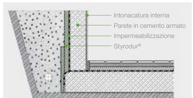
Fig. 18: Punto inferiore dell'isolamento perimetrale. La lastra di Styrodur® è posizionata verticalmente sulle fondamenta.
