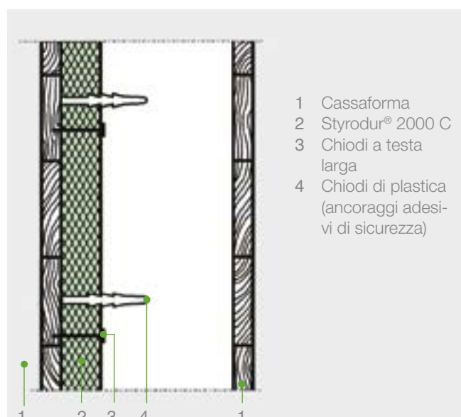
Fig. 13: Fissaggio di lastre di Styrodur® 2000 C alla cassaforma di legno con chiodi a testa larga e ancoraggi adesivi (chiodi di plastica) per l'ancoraggio nel calcestruzzo in casi critici.
