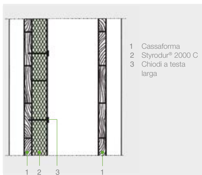
Fig. 12: Fissaggio di lastre di Styrodur® 2000 C alla cassaforma di legno con chiodi a testa larga.
