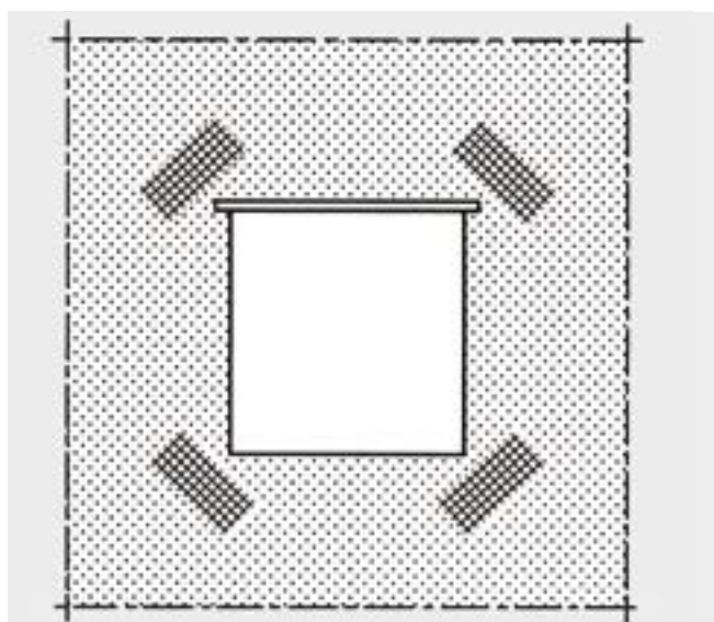
Fig. 23: Armatura diagonale supplementare sugli spigoli della finestra.
