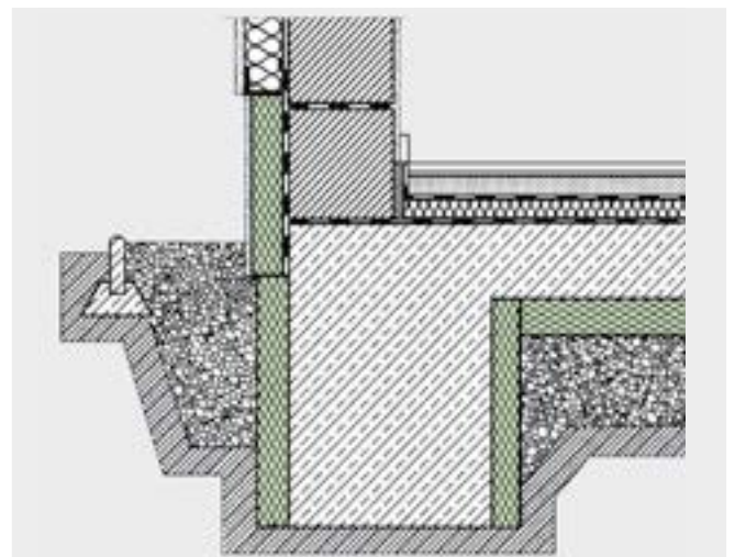
Fig. 11: Isolamento delle fondamenta e raccordo al sistema isolante a cappotto esterno.
