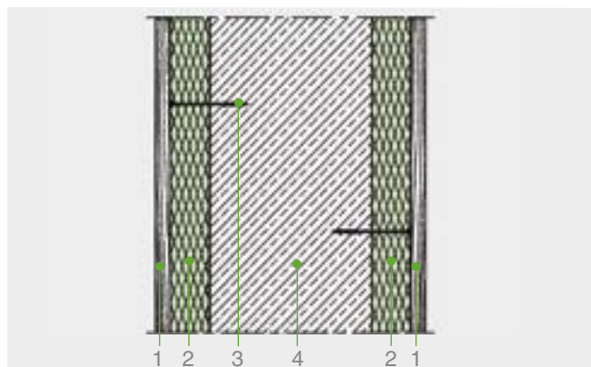
1 Cassaforma 2 Lastra di Styrodur® 3 Chiodi 4 Calcestruzzo
